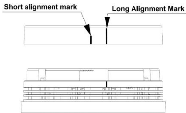
Fig. 6 – Jutiklio tvirtinimas prie bazės
