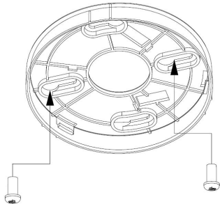
Fig. 5 – Bazės montavimas
